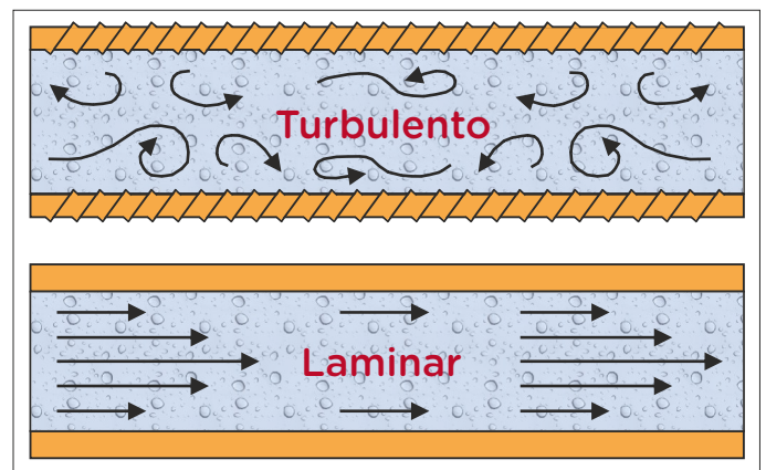
Flujo turbulento vs. laminar. El flujo turbulento aumenta el intercambio de calor; como resultado remueve más calor de la nacedora.
