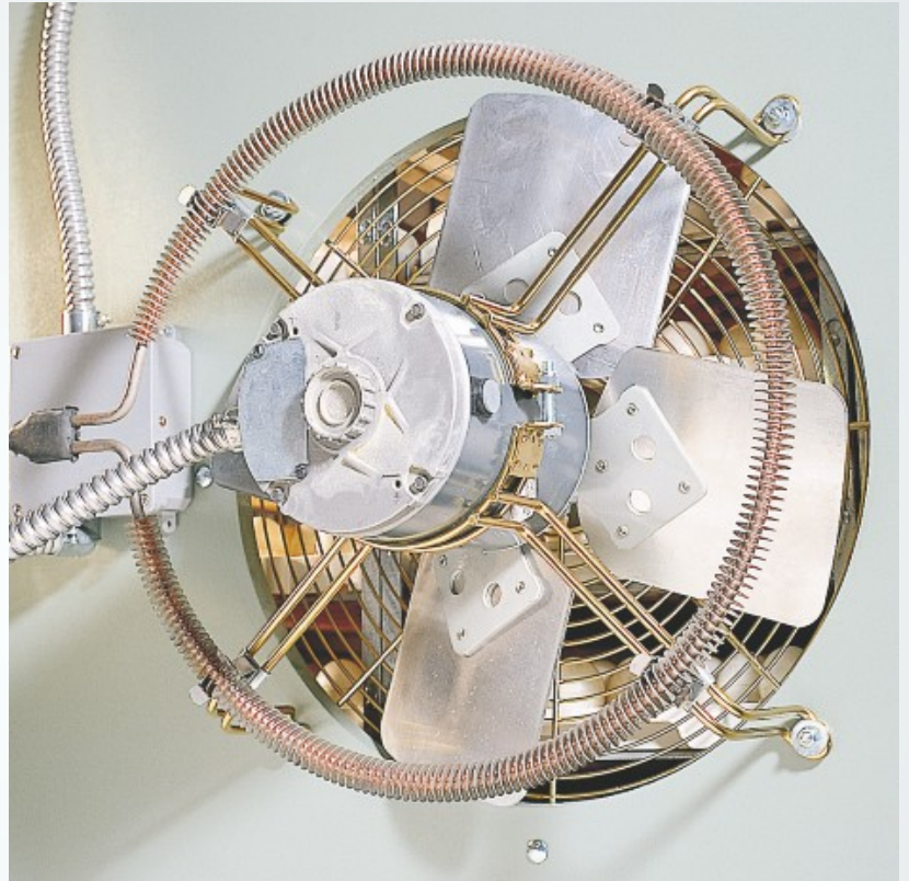
Nuevo elemento de calefacción montado en el ventilador
