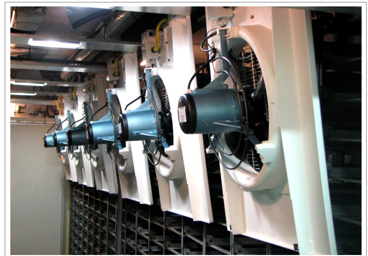
Resistencia de calefacción y sistema de humedad Cyclomist montados en el ensamble del tablero plástico de ventiladores
